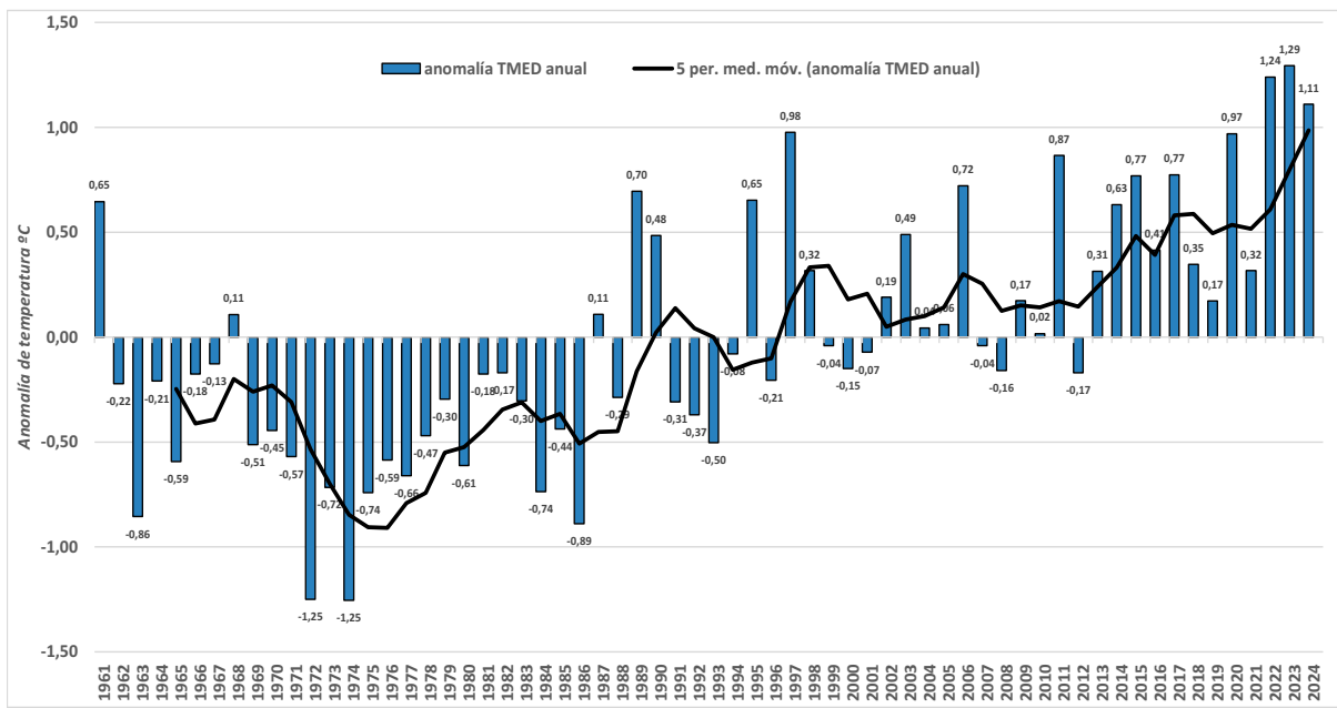
Anomalías de temperatura media no período 1961-2024
