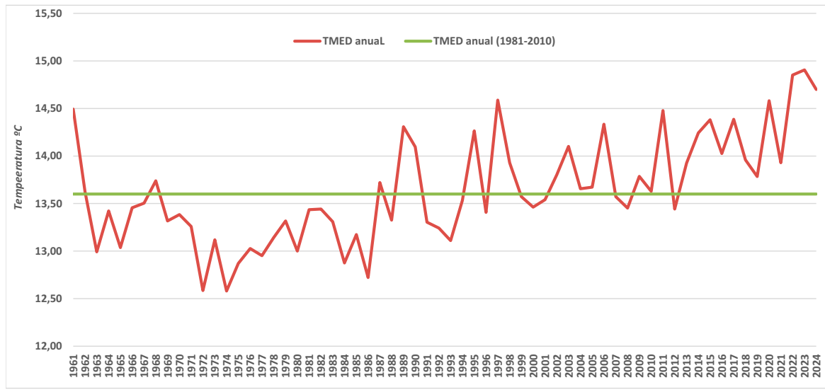
Temperatura media anual no período 1961-2024
