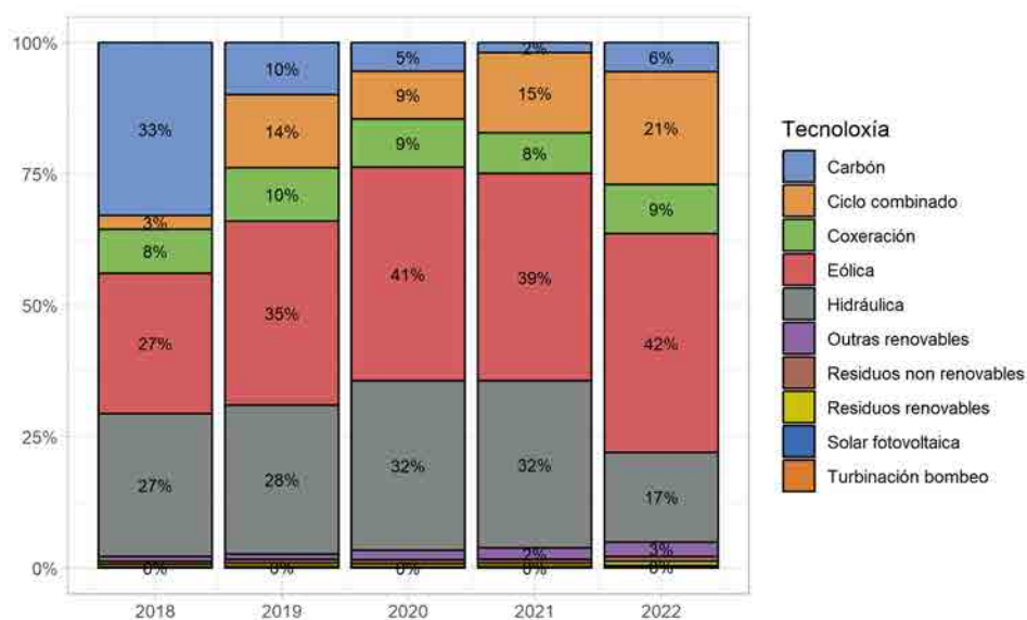
Figura 2.12: Mix de xeración de electricidade por tecnoloxías. Galicia. 2018-2022. Fonte: REE (2022f)
