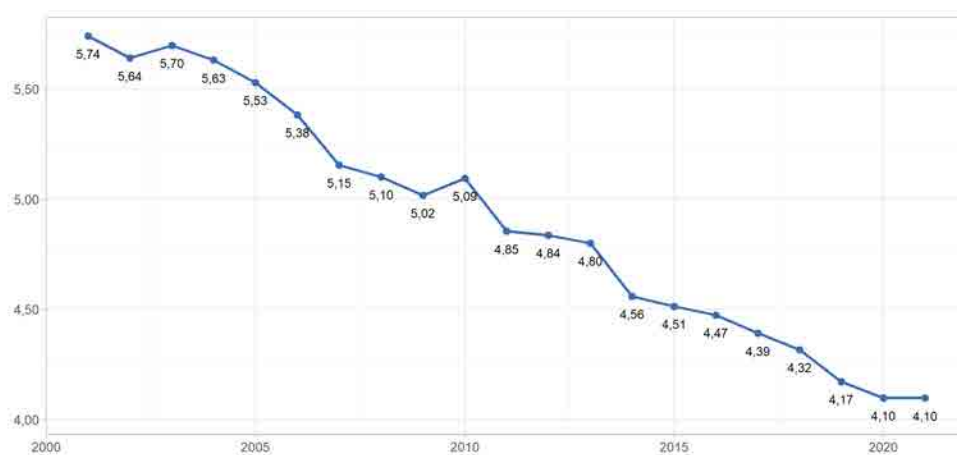
Figura 1.12: Intensidade enerxética primaria Unión Europea. EJ/billón dólares (2015). Fonte: Elaboración propia a partir de BP (2022) e World Bank (2022)
