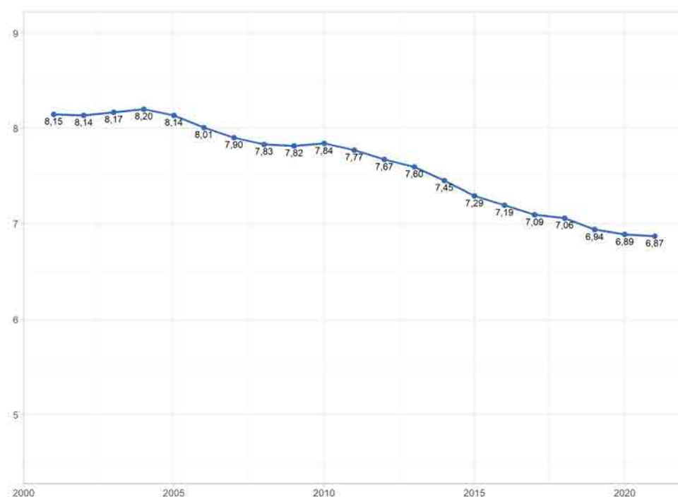
Figura 1.5: Intensidade enerxética primaria mundial. EJ/billón dólares (2015). Fonte: Elaboración propia a partir de BP (2022) e World Bank (2022)
