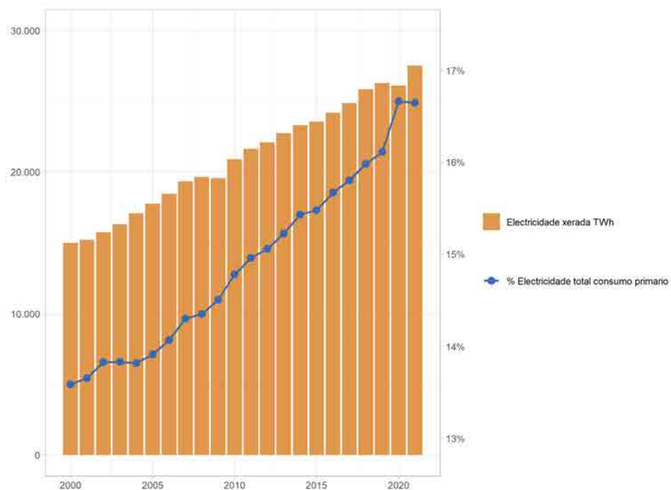
Figura 1.7: Electricidade xerada a nivel mundial (eixo esquerdo). Porcentaxe de electricidade sobre consumo primario de enerxía (eixo dereito). Fonte: elaboración propia a partir de EMBER (2022)
