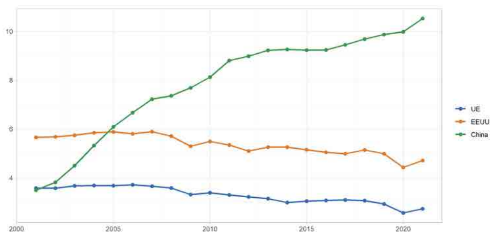
Figura 1.11: Emisións CO 2 (GtCO 2 ) da UE-27, EE. UU. e China. Fonte: Elaboración propia a partir de BP (2022)
