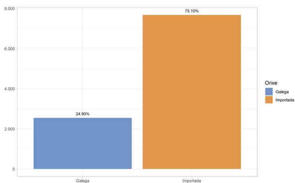
Figura 2.3: Mix de enerxía primaria: enerxía autóctona e enerxía importada. Galicia. Ano 2019. Fonte: Elaboración propia a partir de datos de INEGA (2021a)
