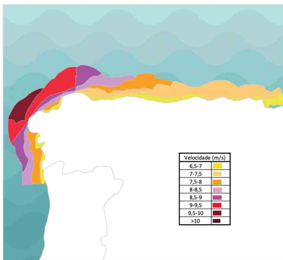
Figura 2.25: Potencial Eólico Mariño na demarcación Noratlántica. Fonte: MITECO-Folla de Ruta para a Eólica Mariña e as Enerxías do Mar (MITERD 2021c).
