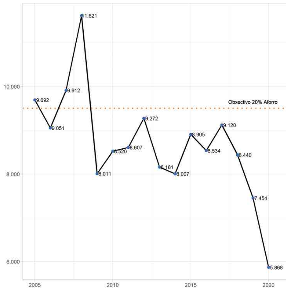
Figura 2.9: Consumo de enerxía primaria e obxectivo do 20 % de aforro enerxético proposto. Fonte: INEGA (2021d)
