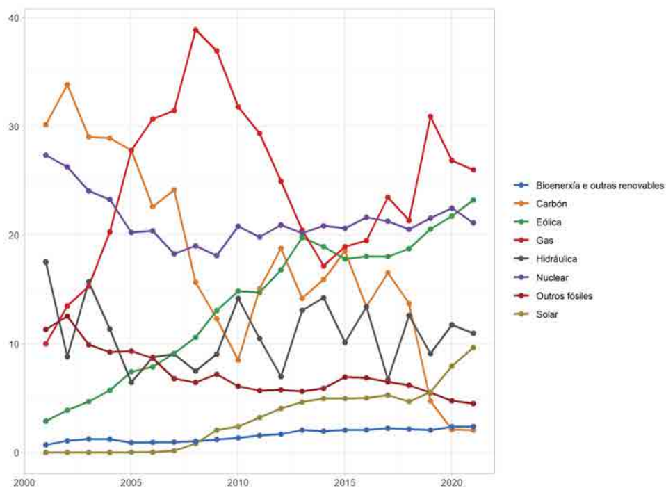
Figura 1.24: Participación dos recursos primarios na xeración de electricidade en España. Fonte: elaboración propia a partir de EMBER (2022)
