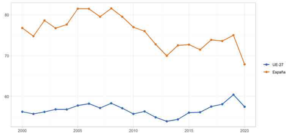
Figura 1.18: Dependencia enerxética España e UE-27 (%). Fonte: elaboración propia a partir de Eurostat (2022a)
