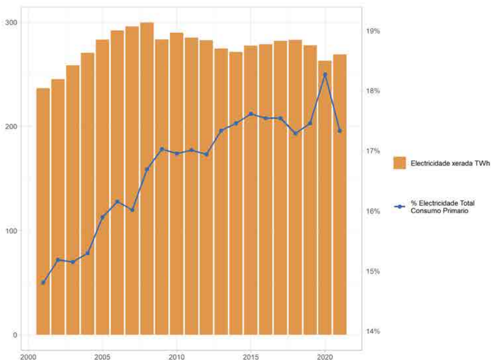
Figura 1.23: Electricidade xerada en España (eixo esquerdo). Porcentaxe de electricidade sobre consumo primario de enerxía (eixo dereito). Fonte: elaboración propia a partir de EMBER (2022)
