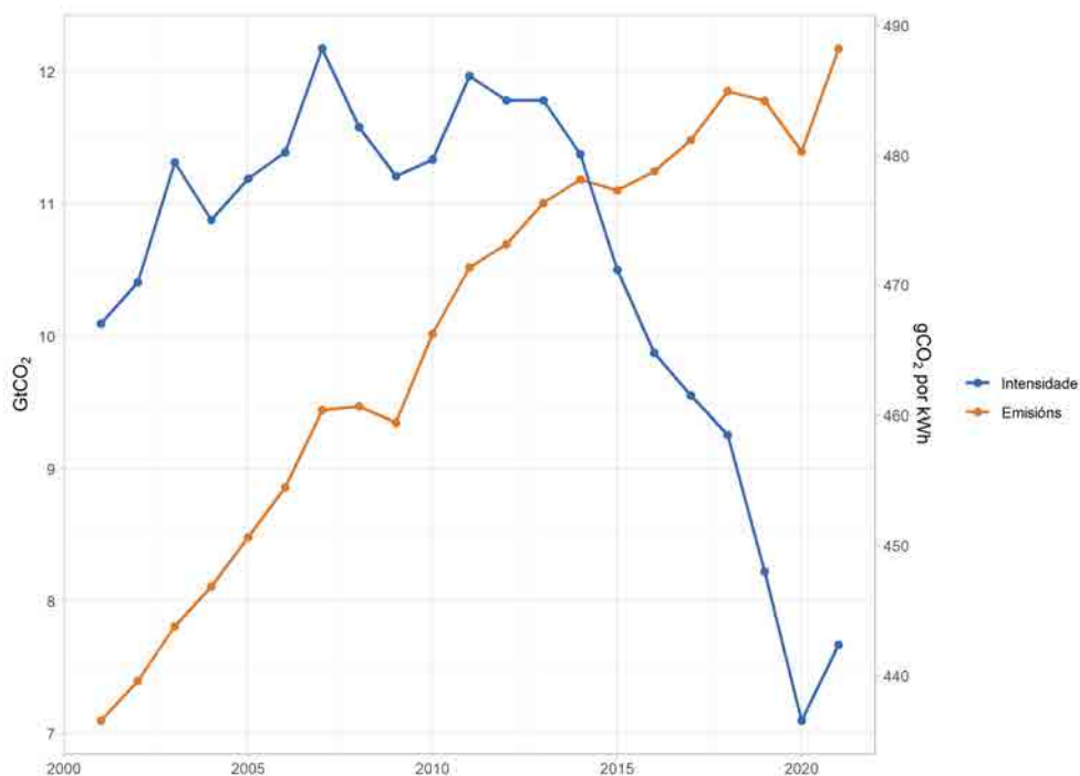
Figura 1.9: Emisións mundiais asociadas á xeración de electricidade (eixo esquerdo). Intensidade das emisións por electricidade xerada (eixo dereito). Fonte: Elaboración propia a partir de EMBER (2022)
