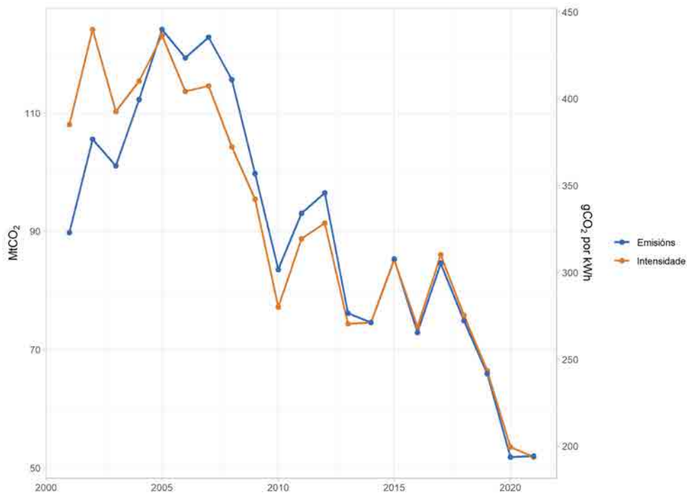
Figura 1.25: Emisións en España asociadas á xeración de electricidade (eixo dereito). Intensidade das emisións por electricidade xerada (eixo esquerdo). Fonte: elaboración propia a partir de EMBER (2022)
