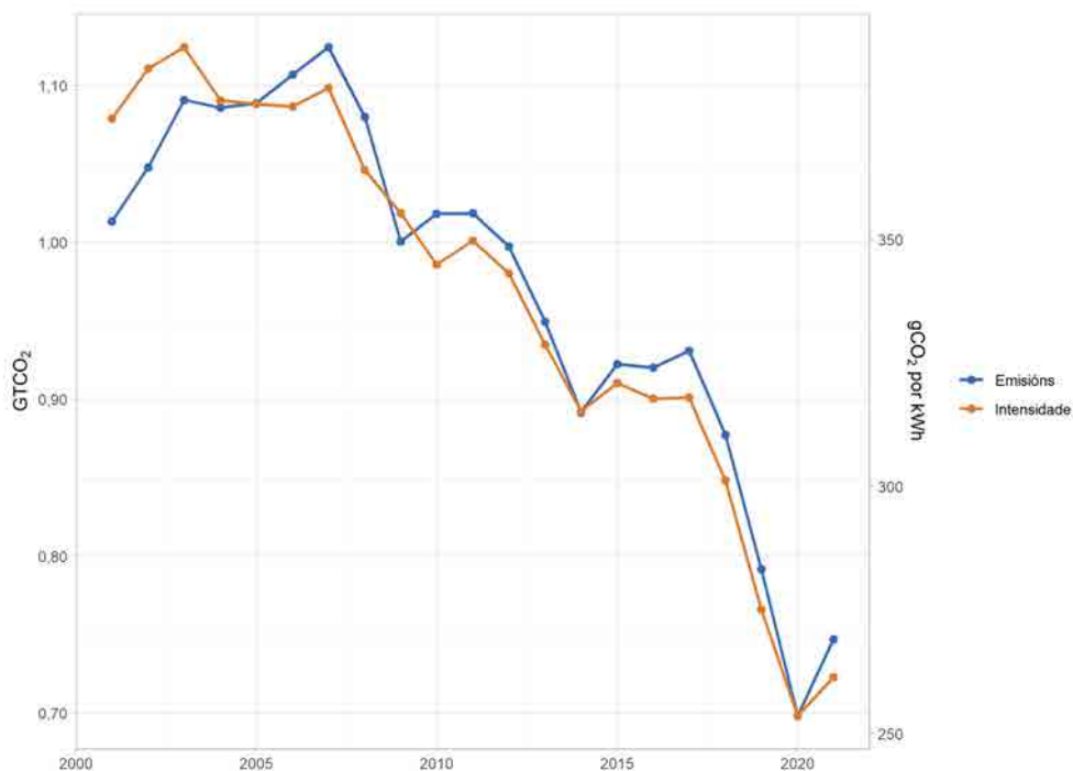
Figura 1.17: Emisións da UE-27 asociadas á xeración de electricidade en GtCO 2 (eixo esquerdo). Intensidade das emisións por electricidade xerada en gCO 2 por kWh (eixo dereito). Fonte: elaboración propia a partir de EMBER (2022)
