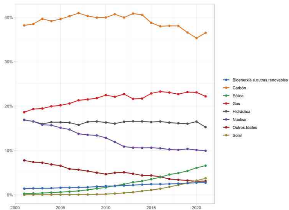
Figura 1.8: Participación dos recursos primarios na xeración de electricidade a nivel mundial. Fonte: elaboración propia a partir de EMBER (2022)
