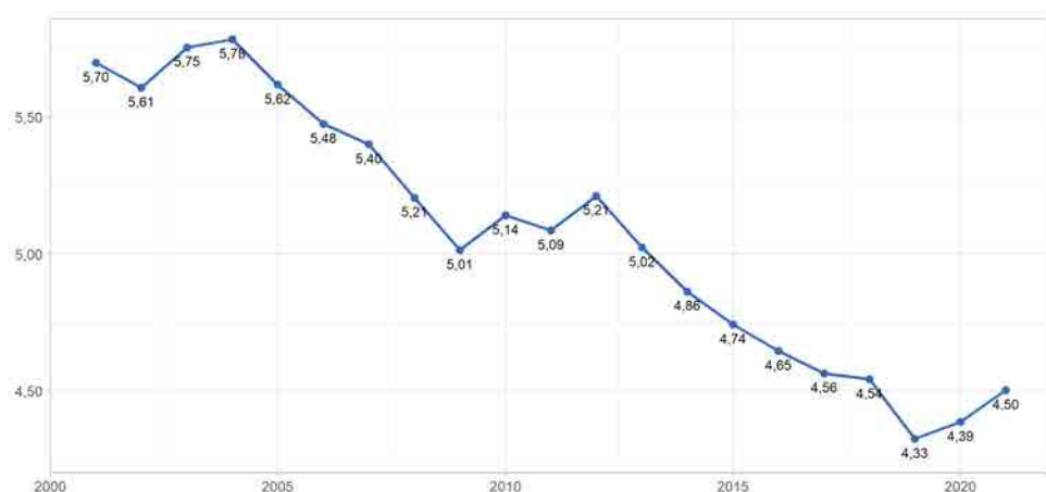
Figura 1.21: Intensidad energética primaria española. EJ/billón dólares (2015). Fuente: elaboración propia a partir de BP (2022) e World Bank (2022)
