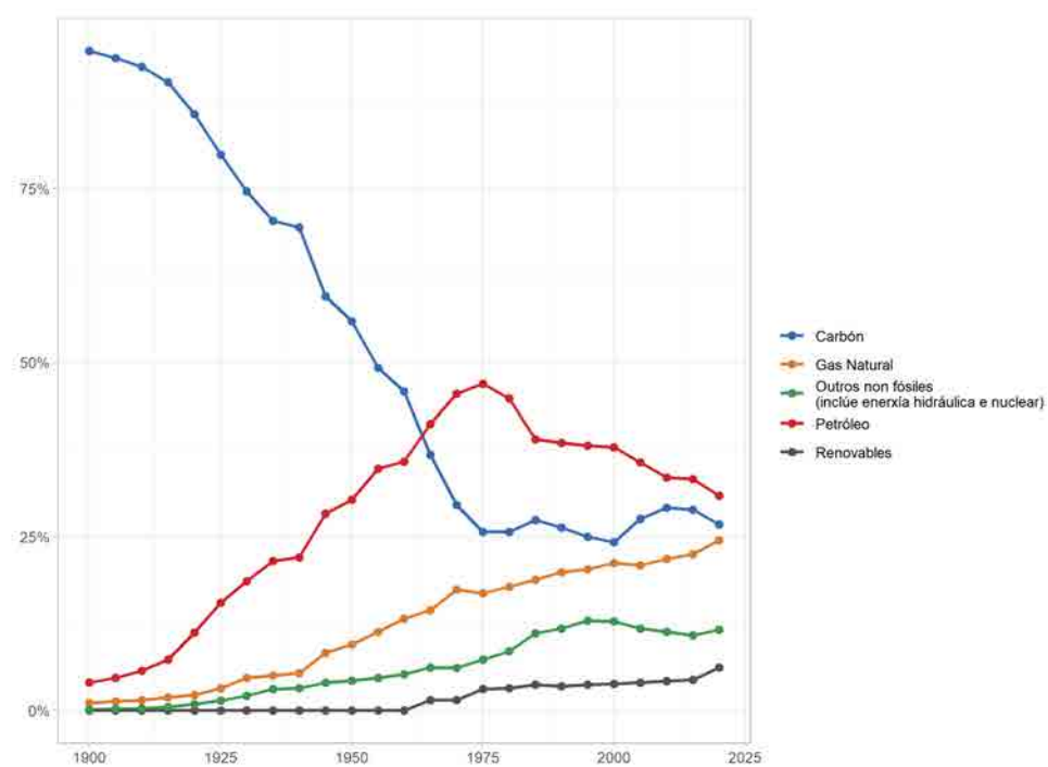
Figura 1.6: Contribución porcentual de recursos primarios ao mix mundial. Fonte: elaboración propia a partir de BP (2022)
