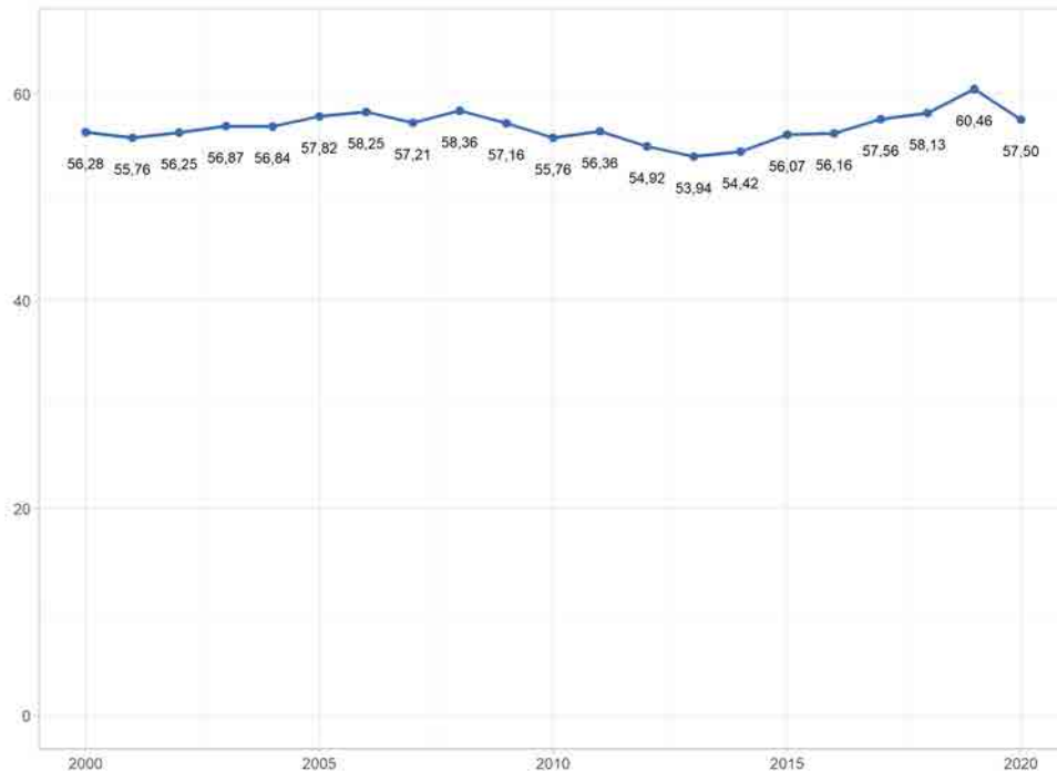
Figura 1.14: Dependencia enerxética UE-27 (%). Fonte: Elaboración propia a partir de Eurostat (2022a)
