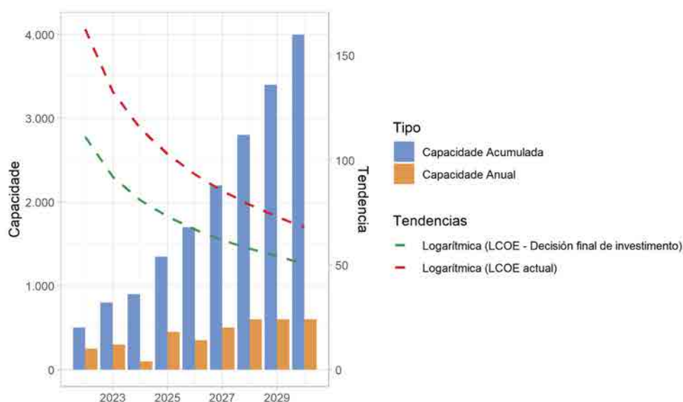
Figura 2.24: Redución do LCOE da eólica flotante ate o 2030. Fonte: Folla de Ruta para a Eólica Mariña e as Enerxías do Mar (MITERD 2021c).
