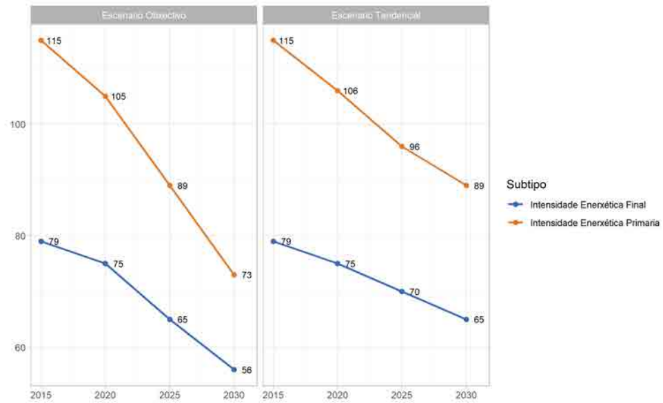
Figura 2.8: Intensidades enerxéticas de enerxía primaria e final nos escenarios tendencial e obxectivo (tep/M€base 2016). Fonte: Plan Nacional Integrado de Enerxía y Clima 2021-2030. MITERD (2020c)
