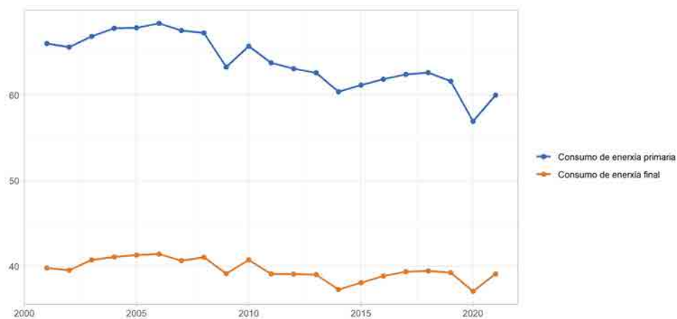
Figura 1.10: Consumo enerxía primaria e enerxía final na UE-27. EJ. Fonte: Elaboración propia a partir de BP (2022) e Eurostat (2022a)
