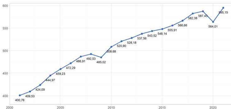
Figura 1.2: Consumo mundial de enerxía primaria. EJ. Fonte: elaboración propia a partir de BP (2022)
