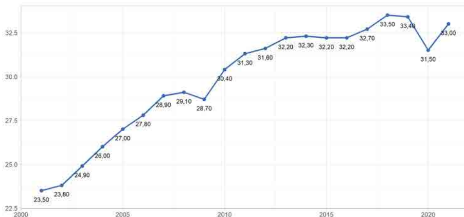
Figura 1.3: Emisións mundiais de CO 2 . Gt. Fonte: elaboración propia a partir de IEA (2022a)
