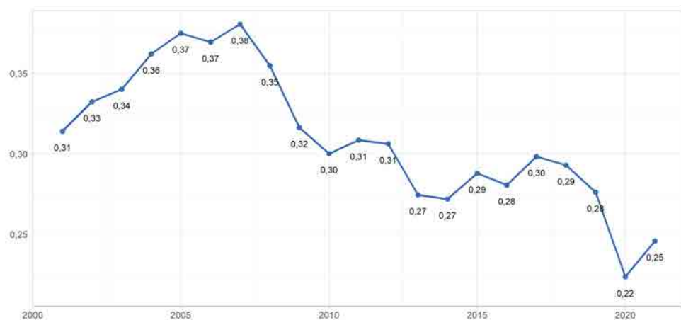
Figura 1.20: . Emisiones españolas CO 2 . Gt. Fuente: elaboración propia a partir de IEA (2022)
