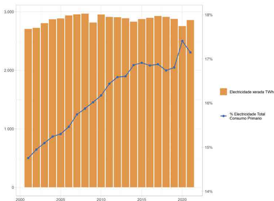
Figura 1.15: Electricidade xerada na UE-27 (eixo esquerdo). Porcentaxe de electricidade sobre consumo primario de enerxía (eixo dereito). Fonte: Elaboración propia a partir de EMBER (2022)
