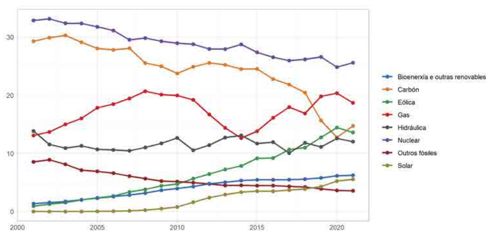
Figura 1.16: Participación dos recursos primarios na xeración de electricidade na UE-27. Fonte: Elaboración propia a partir de EMBER (2022)
