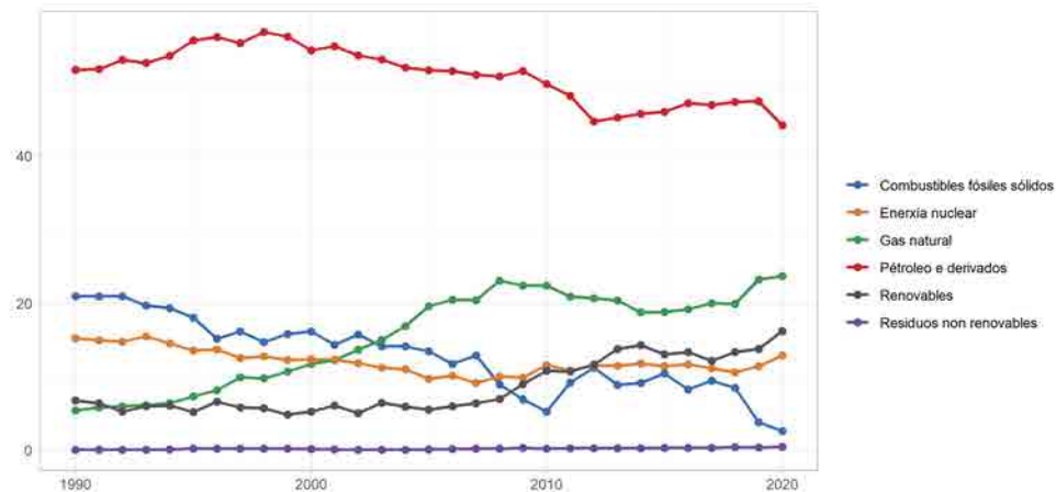
Figura 1.22: Participación porcentual recursos enerxéticos na enerxía bruta dispoñible de España (1990-2020). Fonte: elaboración propia a partir de Eurostat (2022a)
