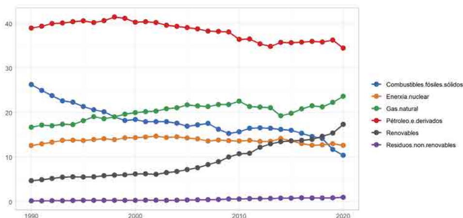
Figura 1.13: Participación porcentual recursos enerxéticos na enerxía bruta dispoñible da UE-27 (1990-2020). Fonte: Elaboración propia a partir de Eurostat (2022a)
