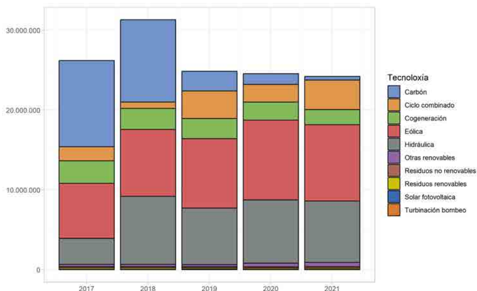
Figura 2.10: Mix de xeración de electricidade por tecnoloxías (MWh). Galicia. 2017-2021. Fonte: REE (2022f)
