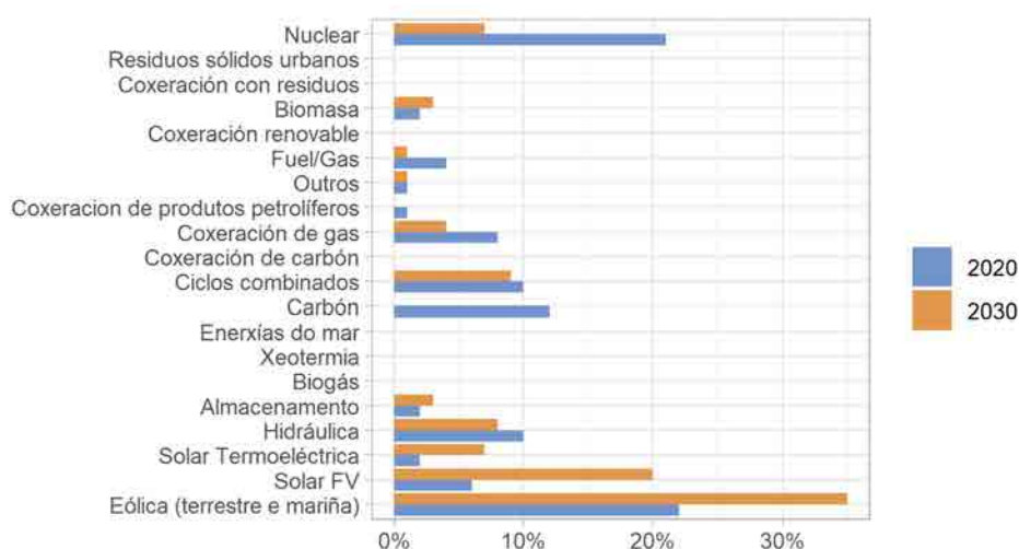
Figura 2.22: Mix de enerxía eléctrica prevista en España. Horizonte 2030. Fonte: PNIEC (MI-TERD 2020c)
