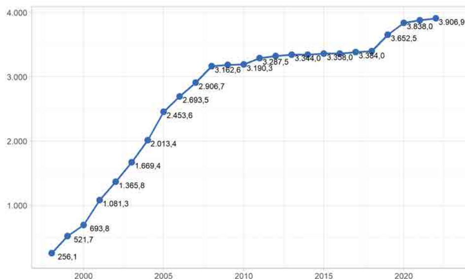
Figura 4.3: MW de potencia eólica instalada en Galicia. Fonte: CNMC (2022f)
