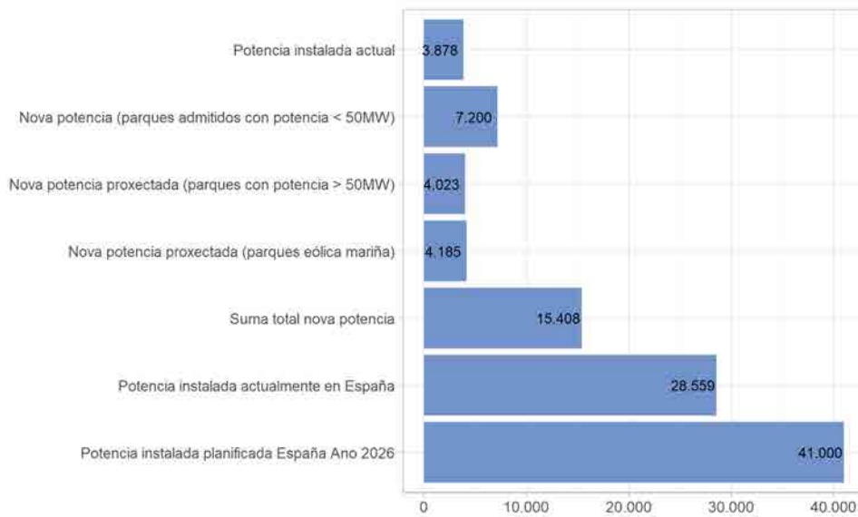
Figura 2.23: Potencia eólica en Galicia (MW) actual e proxectada. Fonte: INEGA (2021a), CCG (2021) e MITERD (2022d)
