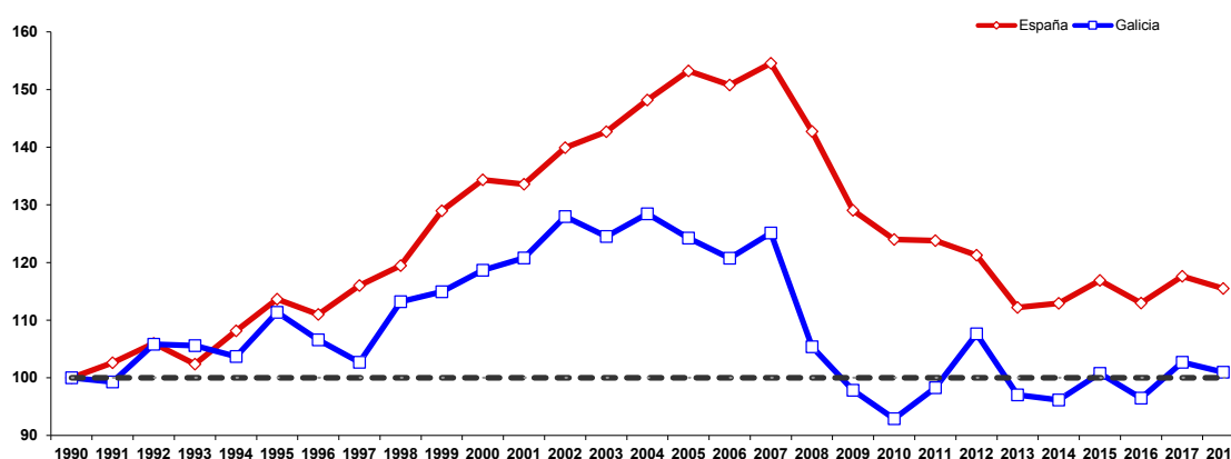
Índice de emisións de CO 2 equivalentes en Galicia e España 1990-2018 (1)
