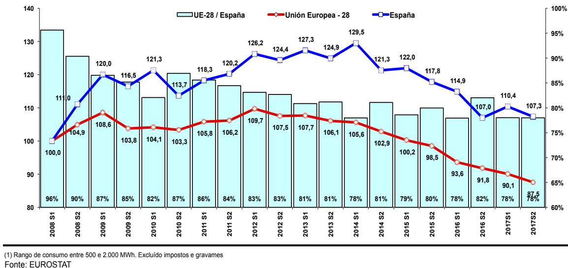
Índices do prezo da electricidade para consumidores industriais na UE-28 e España 2008-17
